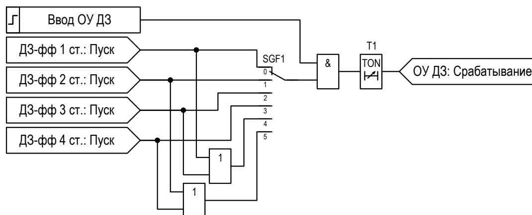
Рисунок 2.10 – Функциональная схема «ОУ ДЗ»
